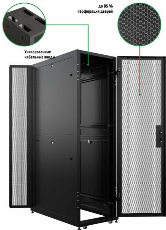
Серверный шкаф «ПРОЦОД»: серии DS и PC
