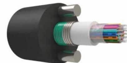
КАБЕЛЬ ОПТИЧЕСКИЙ В КАНАЛИЗАЦИЮ С ЦТ, ПЕРИФЕРИЙНЫЕ СИЛОВЫЕ ЭЛЕМЕНТЫ СТАЛЬНАЯ ПРОВОЛОКА, БРОНИРОВАННЫЙ СТАЛЬНОЙ ЛЕНТОЙ
