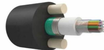
КАБЕЛЬ ОПТИЧЕСКИЙ В КАНАЛИЗАЦИЮ С ЦТ, ПЕРИФЕРИЙНЫЕ СИЛОВЫЕ ЭЛЕМЕНТЫ СТЕКЛОПЛАСТИКОВЫЕ ПРУТКИ, БРОНИРОВАННЫЙ СТАЛЬНОЙ ЛЕНТОЙ
